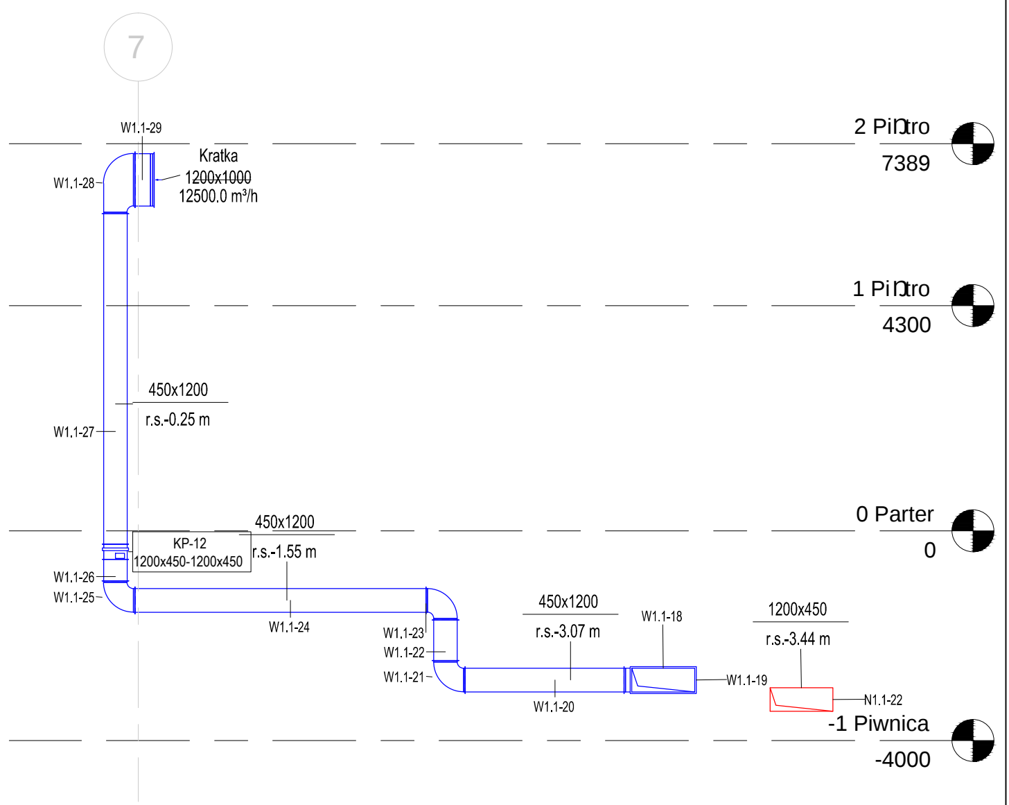
Przekrój B-B
