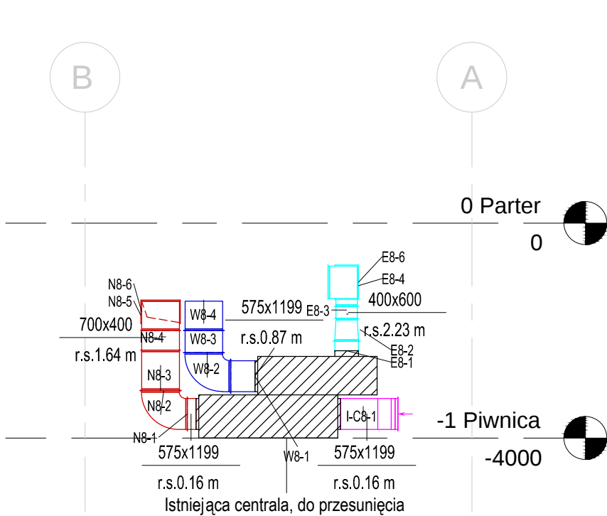
Przekrój B-B
