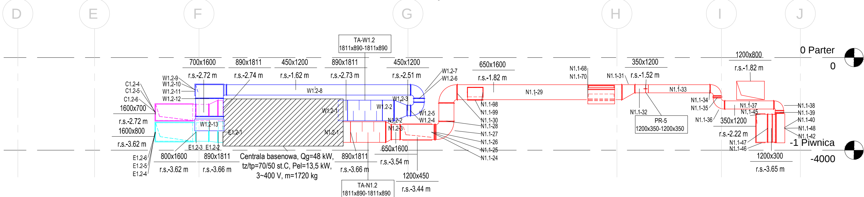
Przekrój C-C
