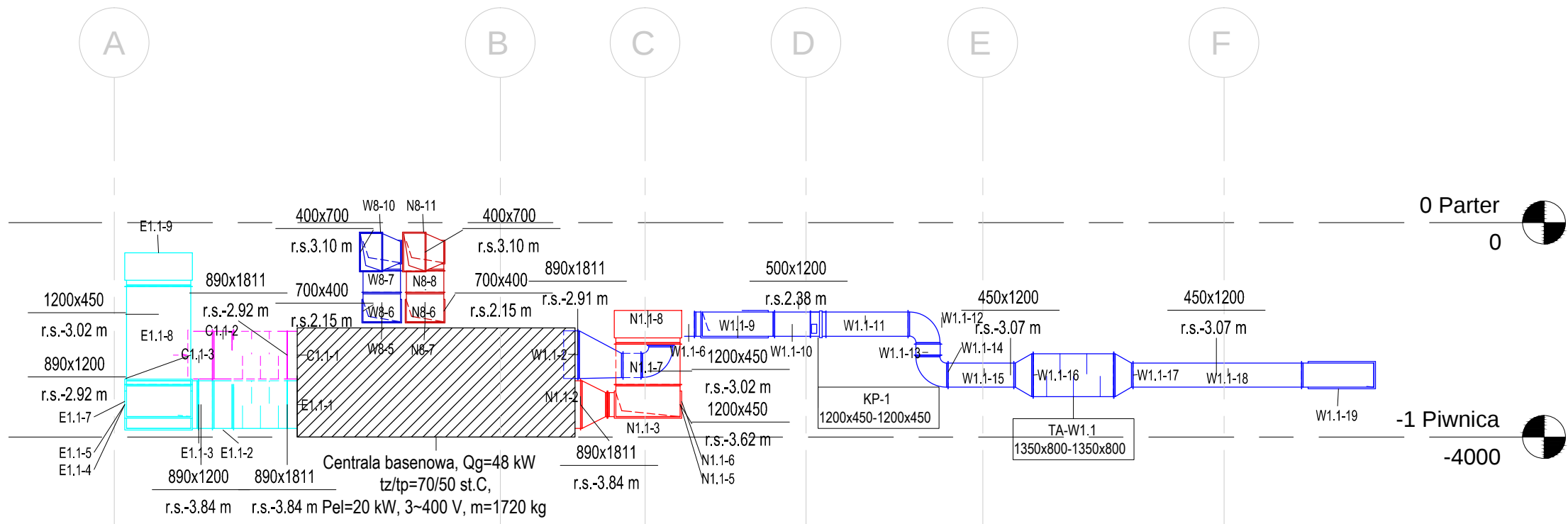
Przekrój C-C
